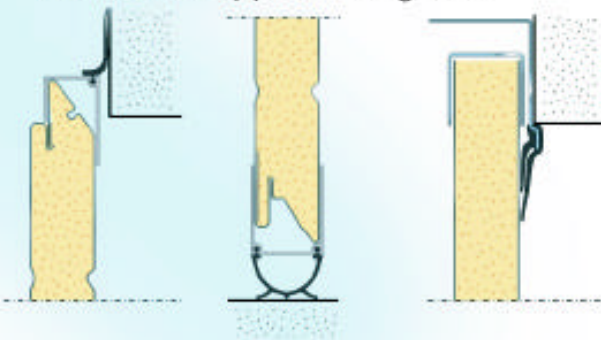
Tettelister i topp, bunn og sider
